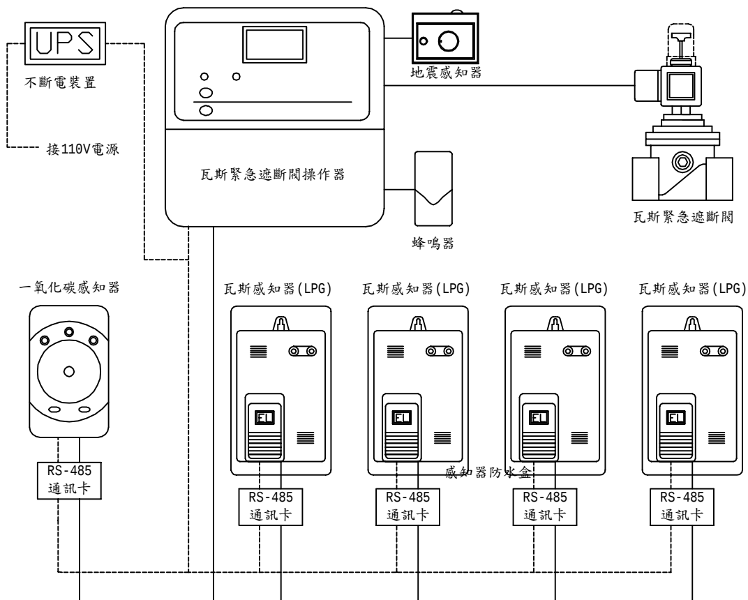
ELS-006瓦斯緊急遮斷系統配備圖(LPG)
