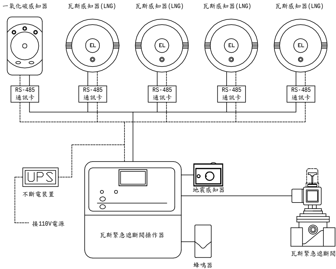
ELS-006瓦斯緊急遮斷系統配備圖(LNG)
